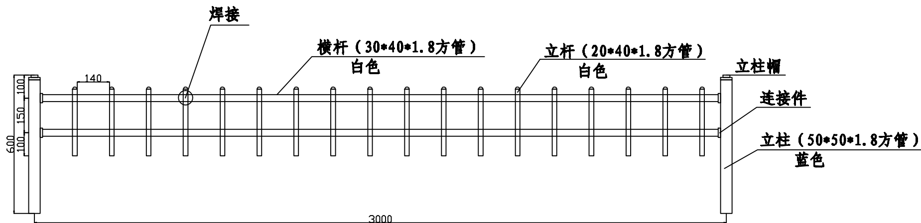
防护栏一 立面图 (单位mm)
